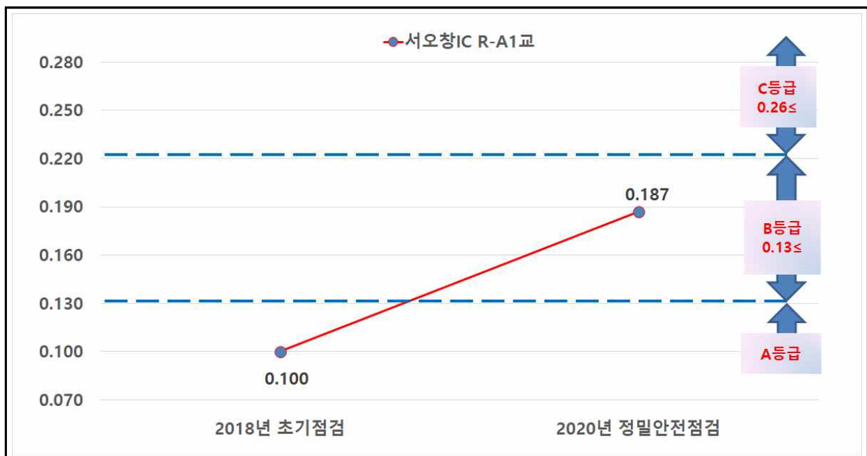
[그림 14.4.1] 서오창IC RAMP-A1교 상태평가 결과 비교 그래프
